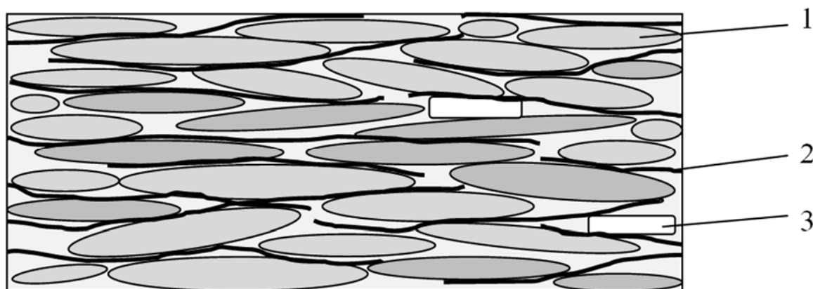
Рис. 2. Конструкция древесно-стружечной плиты: 1 – частицы древесной стружки в смеси с клеем; 2 – волокна осевого слоя в смеси с клеем; 3 – отдельные частицы костры льна в смеси с клеем
