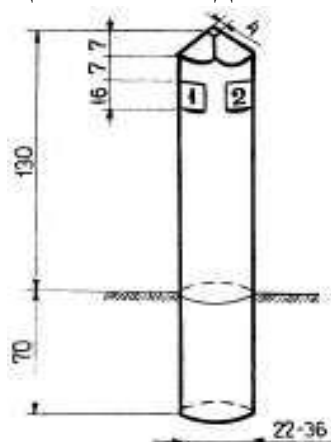
Рис. 137. Квартальный столб
