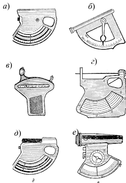
Рис. 106. Высотомеры:
