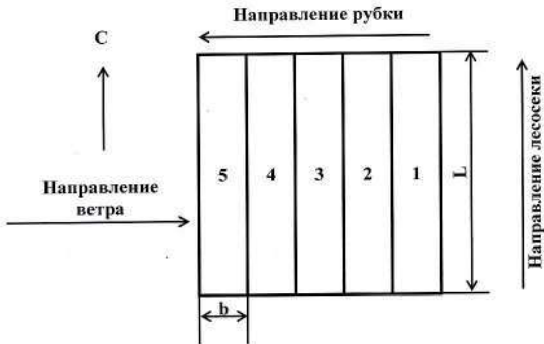
Рис. 50. Схема отвода лесосек:
