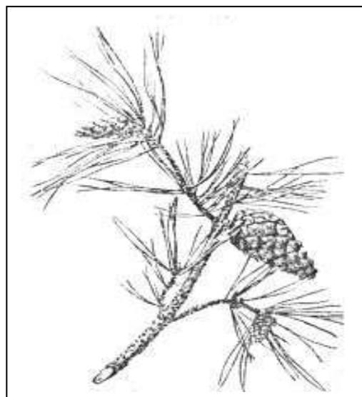
Рис. 8. Сосна обыкновенная
