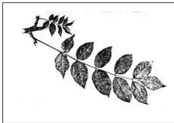
Рис. 17. Ясень обыкновенный
