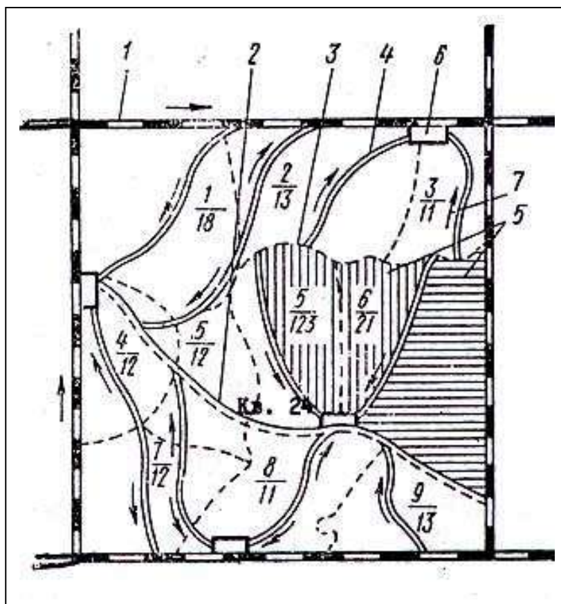
Рис. 69. Схема технологического устройства одного квартала (1x1 км) в блоке: 1 – кварталальная просека, 2 – лесовозная дорога, 3 – граница выдела, 4 – магистральный волок, 5 – пример технологических коридоров, 6 – погрузочная площадка, 7 – направление трелевки (по А.С. Тихонову)
