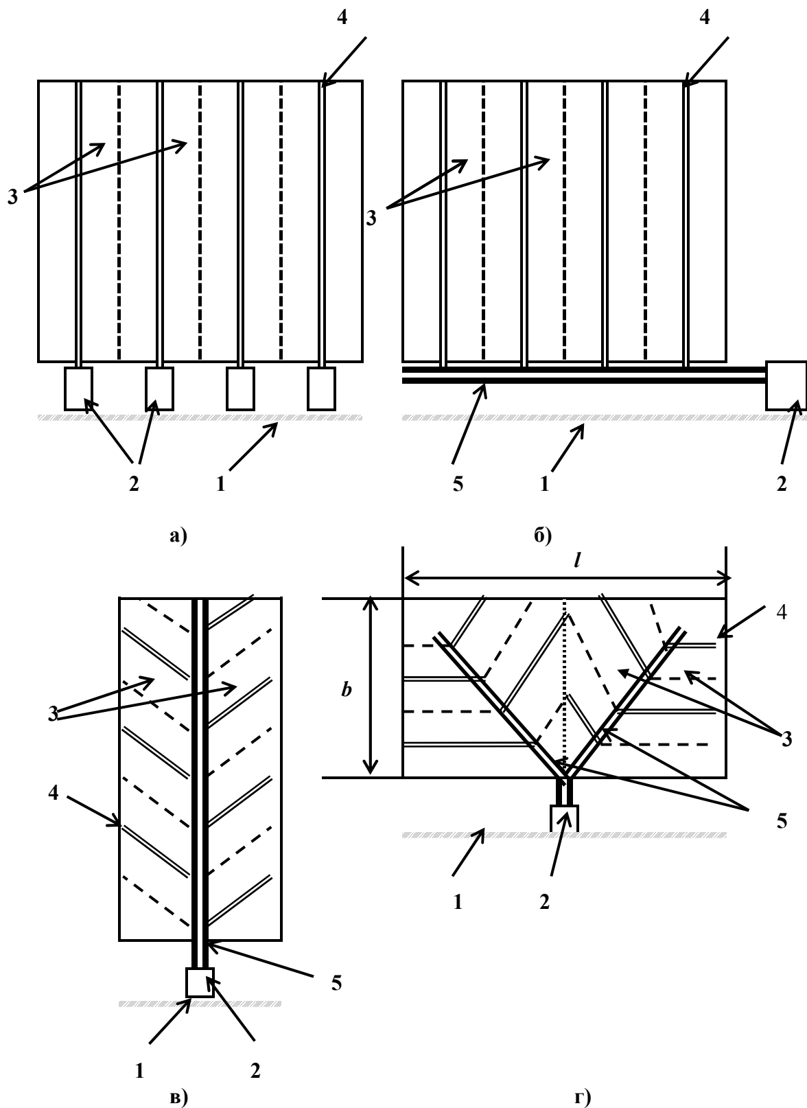
Рис. 53. Типовые схемы размещения волоков: а) метод широкого фронта (параллельная при погрузке широким фронтом); б) параллельная; в) радиальная (веерная); г) диагональная; 1 – лесовозный ус; 2 – погрузочные площадки; 3 – пасаки; 4 – пасечные волоки; 5 – магистральные волоки; l – длина лесосеки; b – ширина лесосеки
