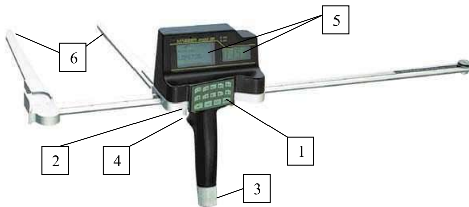
Рис. 103. Мерная вилка Masser 2000:
