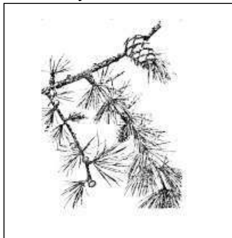
Рис. 11. Лиственница сибирская
