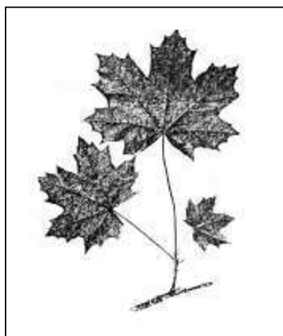
Рис. 18. Клен остролистный
