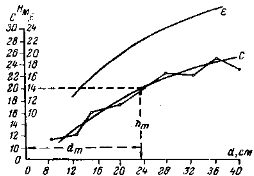
Рис. 136. Графики высот
