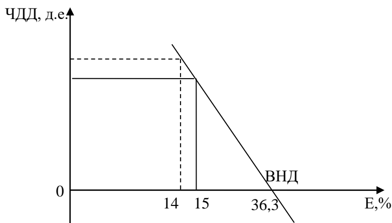
Рис.1. Графический метод нахождения ВНД
