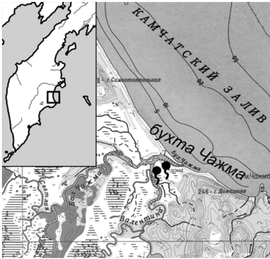
Рис. 1. Географическое положение Нижне-Чажминских термальных источников.
