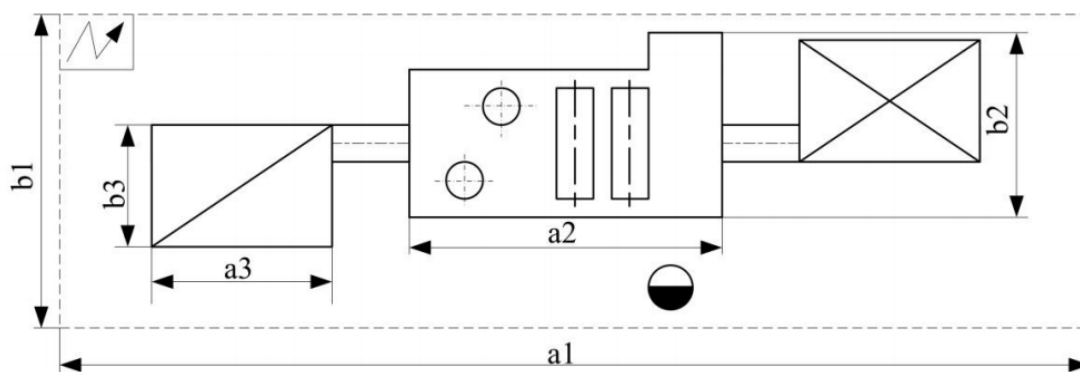
Рис. 2. Схема организации рабочего места многостороннего продольно-фрезерного станка с питателем и накопителем.
