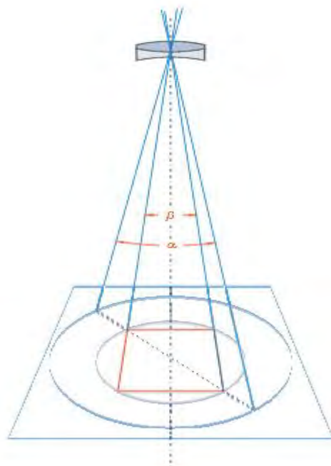
Рис. 1. Угол изображения ( \beta ) и угол зрения ( \alpha ) объектива
