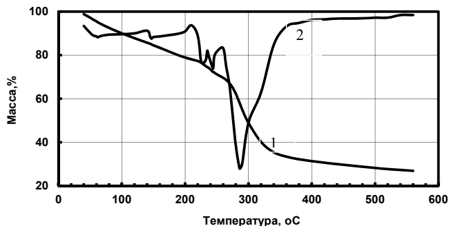
Дериватограмма компонента карбамидоформальдегидной смолы, нерастворимого в воде: 1 – TG; 2 – DTG
