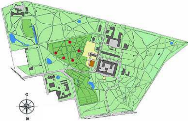
Рис. 3. Схема Ботанического Сада СПбГЛТУ им. С.М. Кирова с расположением устройств Tree Talker
