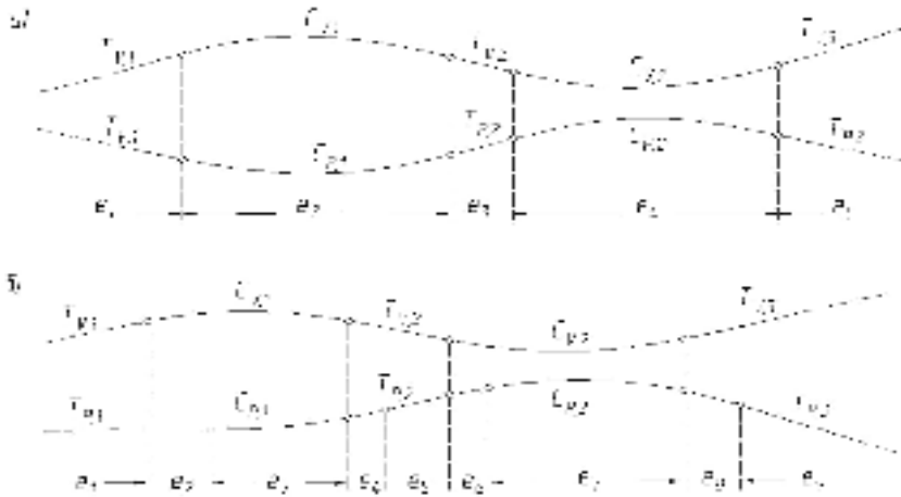
Рис. 2. Варианты сочетания сложных участков плана и продольного профиля
