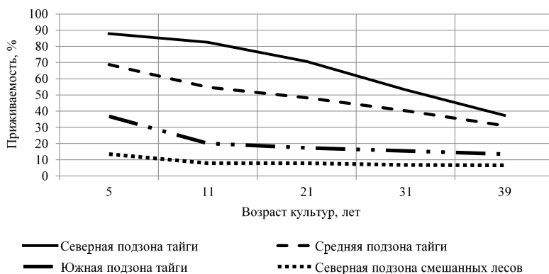
Рис. 1. Динамика приживаемости сосны обыкновенной из различных лесорастительных подзон в географических культурах Архангельской области Fig. 1. Dynamics of survival rate of Scots pine from different forest habitat subzones in geographical cultures of the Arkhangelsk region
