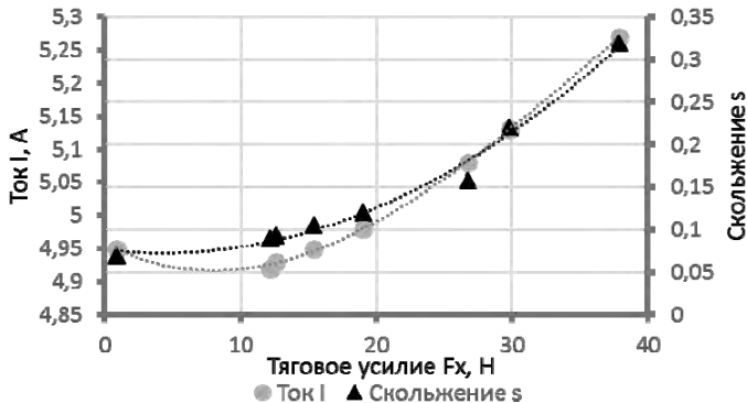
Рис. 3. Рабочие характеристики ЛАДД (зависимости тока и скольжения от тягового усилия, действующего на диск пилы) Fig. 3. Engine performance of LIASM (influence of the tractive effort, acting on the saw blade, on power and frequency)
