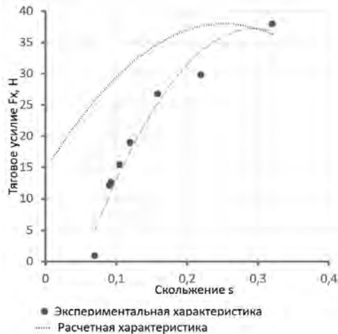
Рис. 6. Механические характеристики ЛАДД F_x = f(s)
