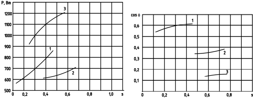
Рис. 8. Зависимости мощности P и \cos \varphi от скольжения s :
