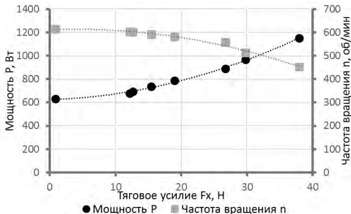
Рис. 4. Рабочие характеристики ЛАДД (зависимости мощности и частоты от тягового усилия)
