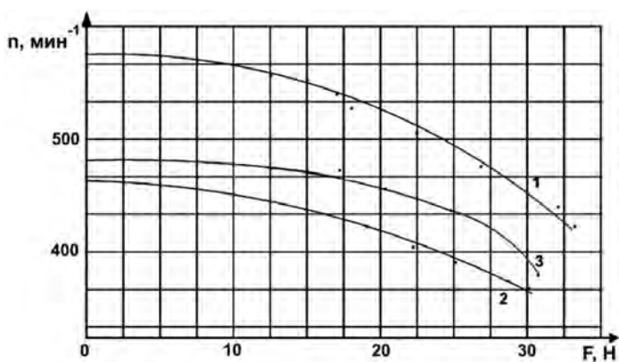
Рис. 7. Механические характеристики ЛАДД:
