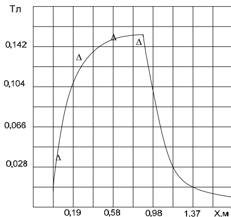
Рис. 9. Экспериментальные ( \Delta ) и расчетные (—) значения магнитной индукции B в воздушном зазоре ЛАДД
