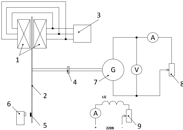
Рис. 2. Электрическая схема экспериментальной установки с ЛАДД для исследования характеристик ЛАДД:
