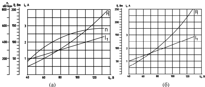
Рис. 5. Характеристики холостого хода (а) и короткого замыкания (б) ЛАДД: P_1 – потребляемая мощность, I_1 – ток статора, n – число оборотов
