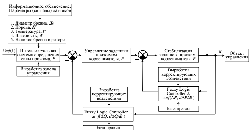
Рис. 2. Разработанная схема интеллектуального управления прижимом короснимателя
