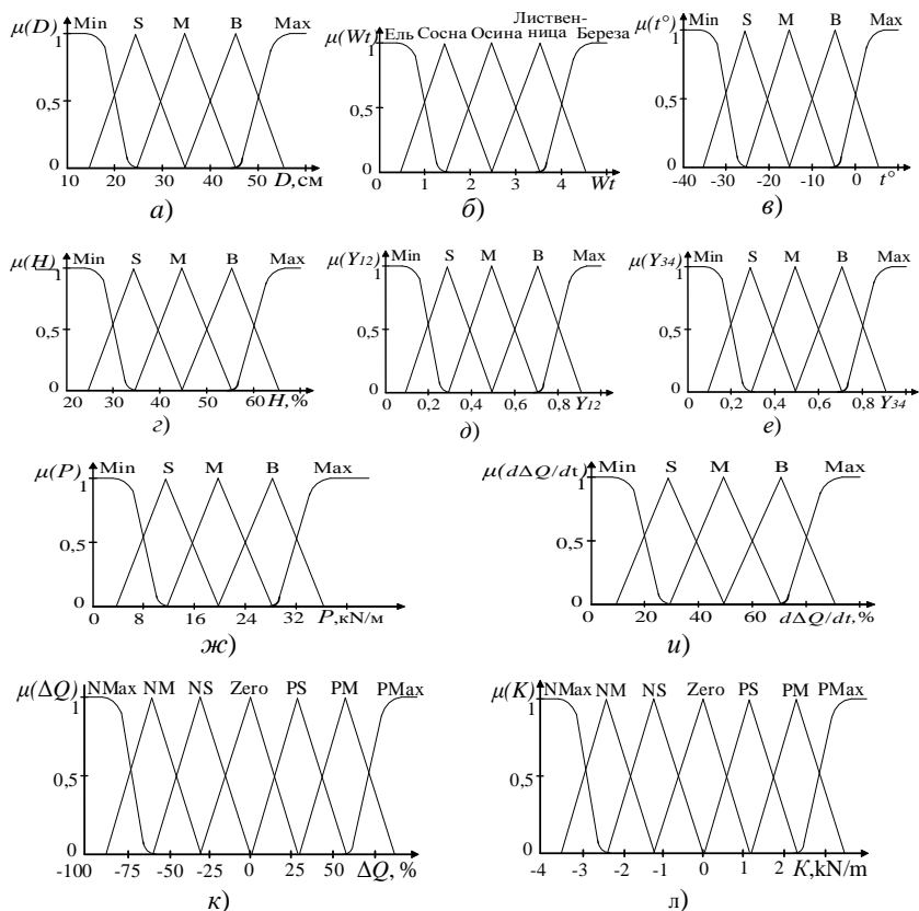
Рис. 4. Лингвистические переменные в задачах нечеткого вывода интеллектуальной системы определения начального прижима и интеллектуальной системы управления прижимом короснимателя: а – переменная «Диаметр бревна, D »; б – «Порода древесины, Wt »; в – «Температура, t^\circ »; г – «Влажность, H »; д – «Температурно-влажностный фактор, Y_{12} »; е – «Породный фактор, Y_{34} »; ж – заданное значение прижима короснимателя «Заданный прижим, P »; и – «Скорость изменения качества окорки, d\Delta Q/dt »; к – «Изменение качества окорки, \Delta Q »; л – «Управление прижимом, K »
