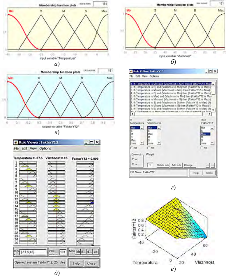
Рис. 5. Нечеткий вывод функции Y_{12} = f(t^{\circ}, H) : а – нечеткая функция принадлежности переменной «Температура, t^{\circ} »; б – нечеткая функция принадлежности переменной «Влажность, H »; в – нечеткая функция принадлежности «Температурно-влажностный фактор, Y_{12} »; г – база правил нечеткого вывода; д – процедура нечеткого вывода и приведения к четкости; е – результирующая функция нечеткого вывода Y_{12} = f(t^{\circ}, H)
