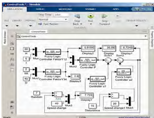
Рис. 7. Программная реализация в Simulink модели интеллектуального управления короснимателем для исследования и настройки нечетких систем Fig. 7. Software implementation in Simulink of the model of intelligent control of the debarking tool for research and tuning of fuzzy systems
