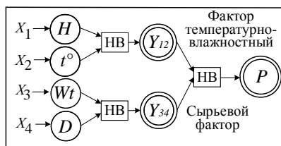
Рис. 3. Обобщенная структура интеллектуальной системы определения начальных значений заданного прижима короснимателей P = f(D, Wt, t^\circ, H) : X1-X4 – входные параметры; НВ-нечеткий вывод
