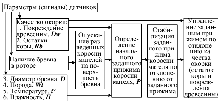
Рис. 1. Схема технологического процесса работы и управления инструмента окорочного станка
