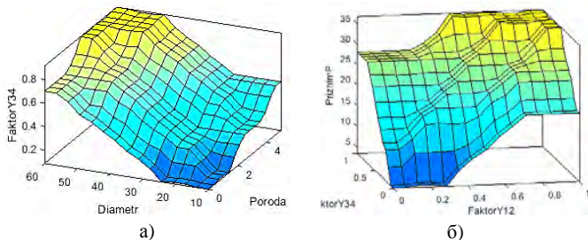
Рис. 6. Графики функций, полученных в результате нечетких выводов: а – «Сырьевой фактор, Y_{34} »; б – «Заданный прижим, P » Fig. 6. Graphs of functions obtained as a result of fuzzy conclusions: а – "Raw material factor, Y_{34} "; б – "Set pressure, P "
